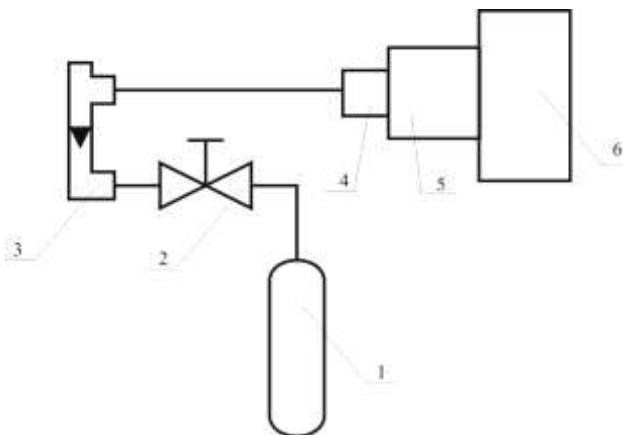
Рисунок А.1 - Схема подачи газовой смеси для проверки
