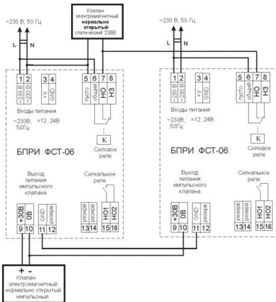
Рисунок. 5.4 Два ФСТ-06 И на один клапан
