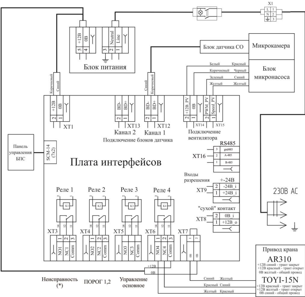
Рисунок 5.3 Монтажная схема БПС ФСТ-07
