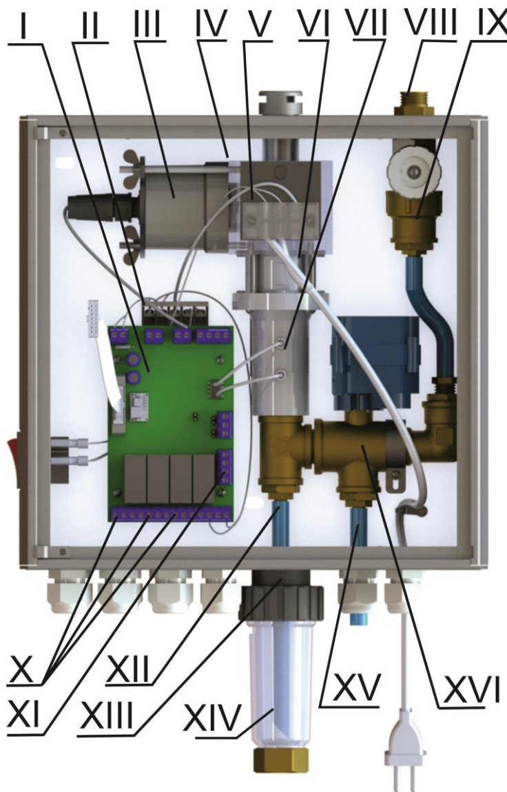
Рисунок 4.1 Вид БПС ФСТ-07 со снятой передней панелью.
