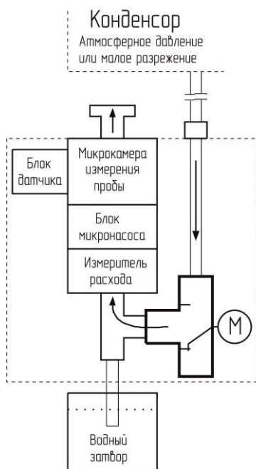
Рисунок 4.4 Тракт при принудительной подаче пробы
