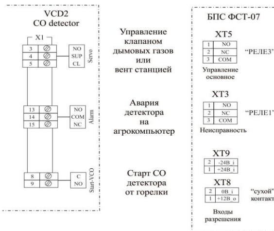
Рисунок 5.7. Соответствие сигналов и контактов VCD2 и ФСТ-07.
