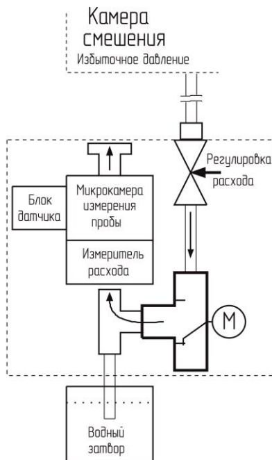
Рисунок 4.5 Тракт подачи пробы при помощи избыточного давления
