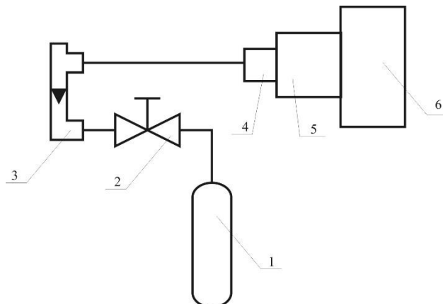
Рисунок А.1 - Схема подачи поверочной газовой смеси
