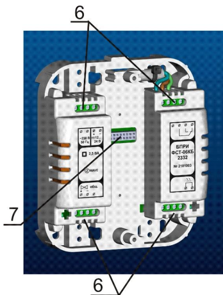
Рисунок 4.1 ФСТ-06 общий вид.
