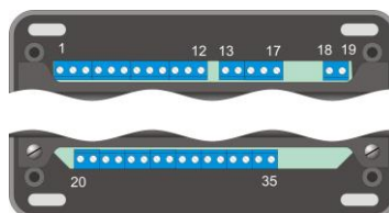
Рисунок 6.3 Клеммы БПС 24В.
