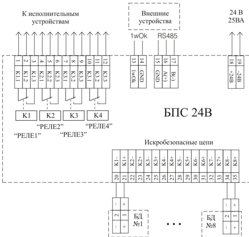
Рисунок 6.5 Монтажная схема БПС 24 В.
