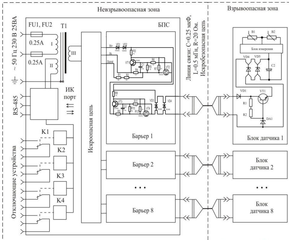
Рисунок 5.1 Средства обеспечения взрывозащищенности БПС 230В
