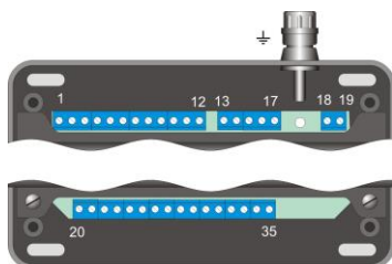
Рисунок 6.2 Клеммы БПС 230В.
