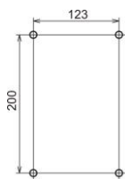
Рисунок 6.1. Разметка для крепления
